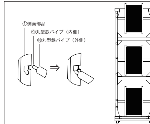
図 2. 丸型鉄パイプ取り付け
