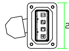
コネクタ方向 負荷側引出し
