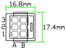
モータ側コネクタ 配線側から見た図
